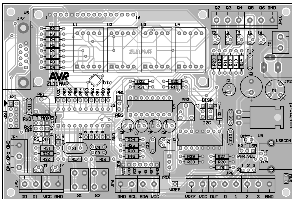
Rys. 4. Schemat montażowy zestawu ZL11AVR
