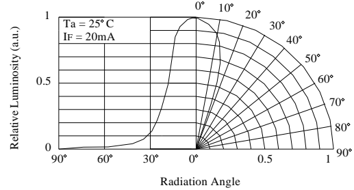
Directivity (Angle : 35^\circ )
