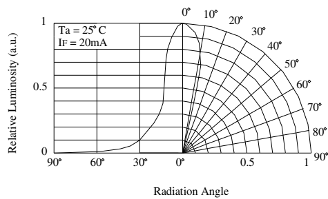
Directivity (Angle : 25°)
