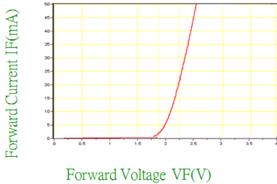
Fig.1 IF-VF(Ta=25°C)
