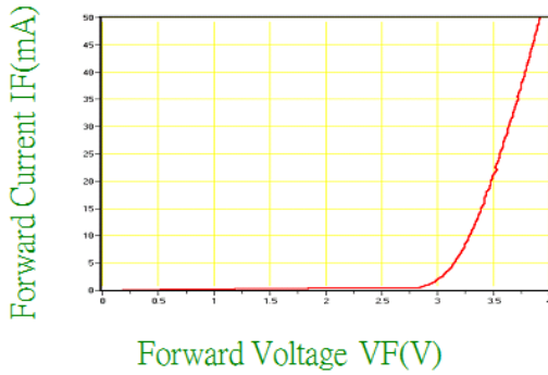
Fig.1 IF-VF(Ta=25°C)
