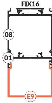
variant 15 - ceiling FIX16-08-01-E9 wariant 15 - sufitowy FIX16-08-01-E9
