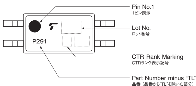
(b) SO4 Package (TLP291)
