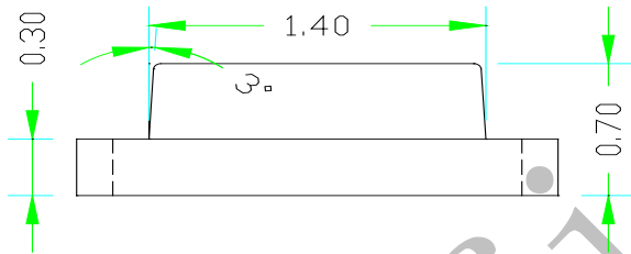
侧面视图
