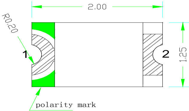
正面视图
