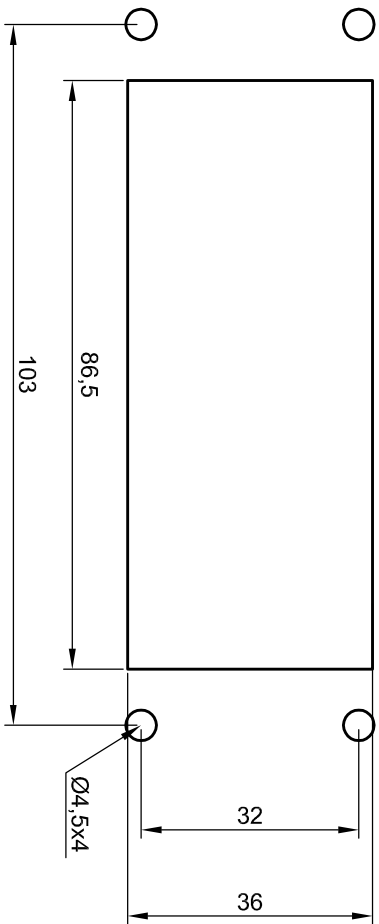
Panel cut out Foratura del pannello
