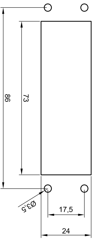
Foratura del pannello Panel cut out
