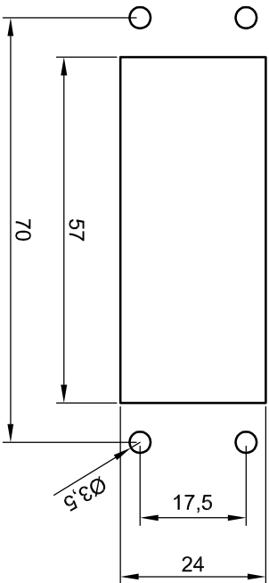
Foratura del pannello Panel cut out
