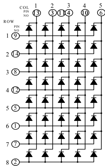
LMD14058BAG-101
