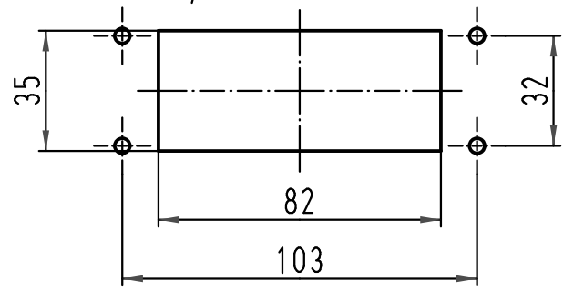
1:2 Montageausschnitt panel cut out
