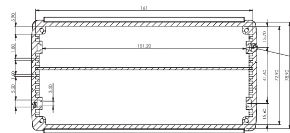
SEZIONE A-A
