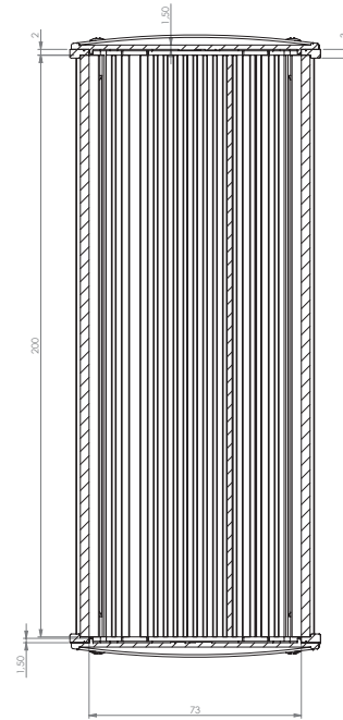
SEZIONE B-B
