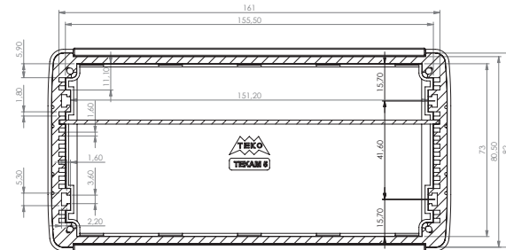
SEZIONE A-A
