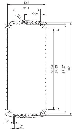
SEZIONE A-A
