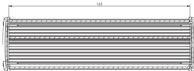
SEZIONE B-B
