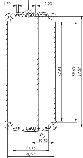
SEZIONE A-A
