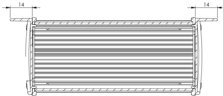
SEZIONE B-B
