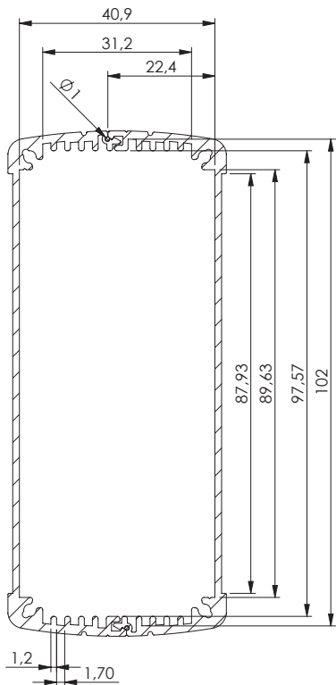
SEZIONE A-A
