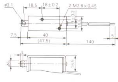
外形寸法 Dimensions
