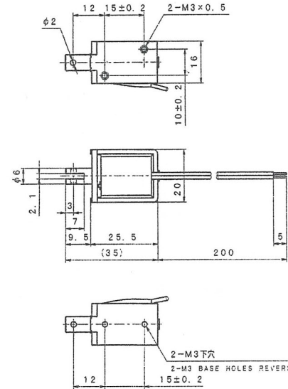
外形寸法 Dimensions
