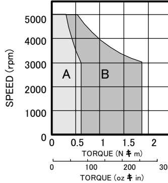
SGMAH-02B
