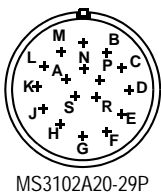
MS3102A20-29P
