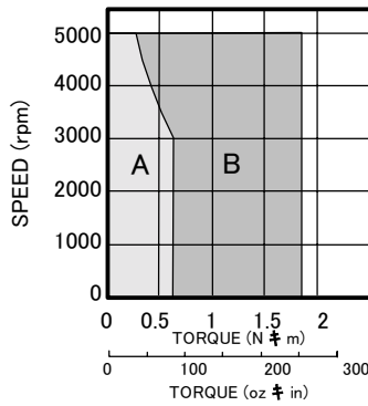
SGMAH-02A
