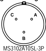
MS3102A10SL-3P
