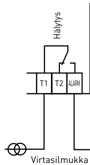
Virtasilmukan kytkentä (lepotila)
