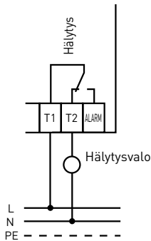
Hälytysvalon (kaavio) tai summerin (lepotila) kytkentä
