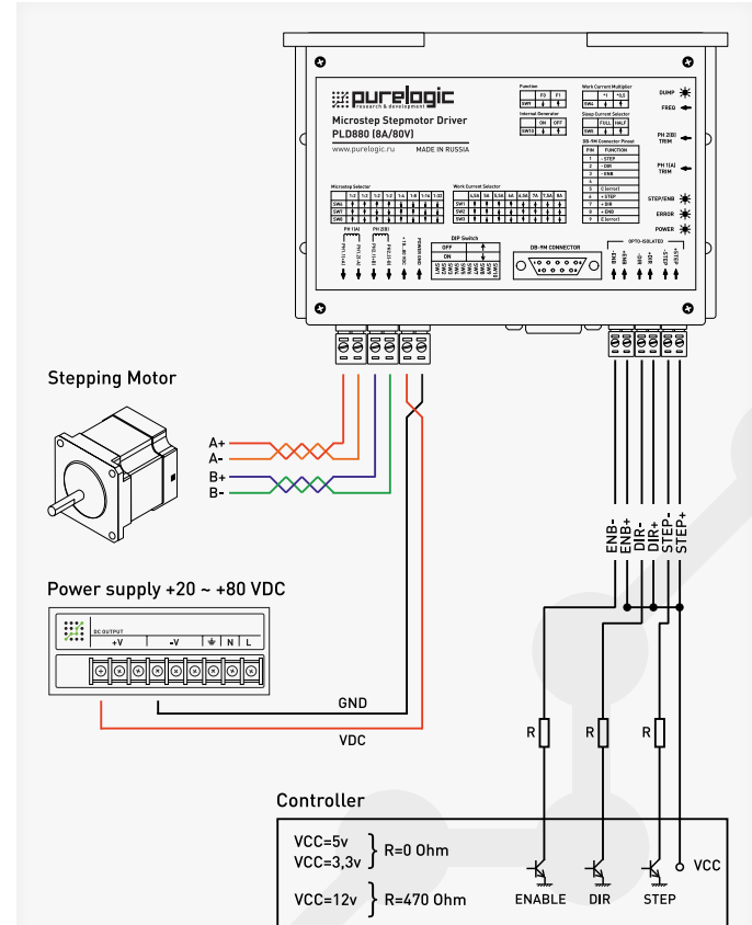
Рис. 5. Схема подключения драйвера ШД
