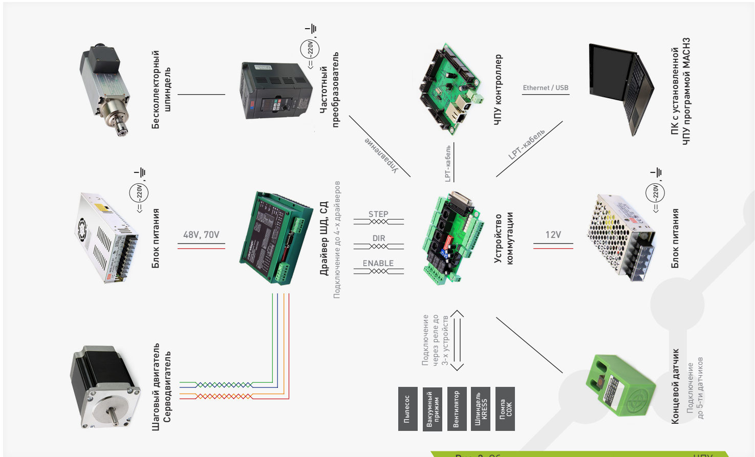
Рис. 3. Общая схема системы управления станком ЧПУ
