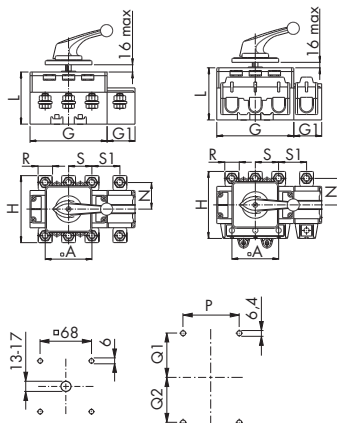
Крепление на основании
