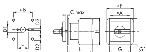
Монтажные отверстия KG10A – KG105C, KF16 – KF63B лицевой панели
