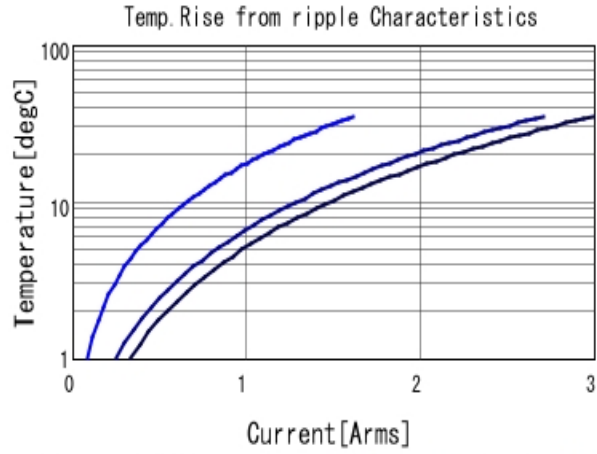
GRM188R71C105KE15 Temp. rise ■ 100kHz ■ 500kHz ■ 1MHz
