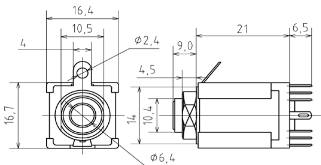
AUB-23 Разъем аудио 1/4" гнездо на приборный блок, стерео, 6 контактов
