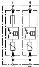
Принципиальная схема DG M TN CI 275
