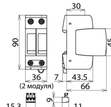
Размерный эскиз DG M TN CI 275
