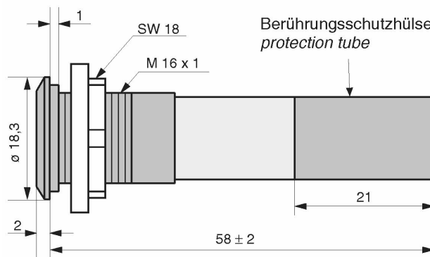
Flachdichtung / gasket
