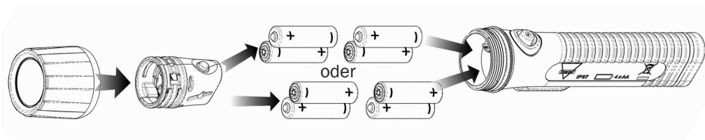
Bild 4: Explosionszeichnung PetaLux Typ 4910... mit Batterien
