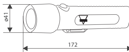
Bild 3: Abmessungen PetaLux Typ 4910...
