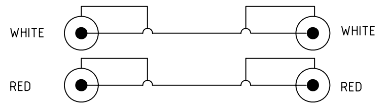
WIRING DIAGRAM RCA PLUG(L) RCA PLUG(R)
