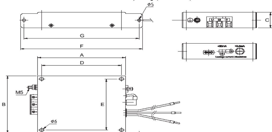
EMV-Filter - Dreiphasig (FPF-8123)
