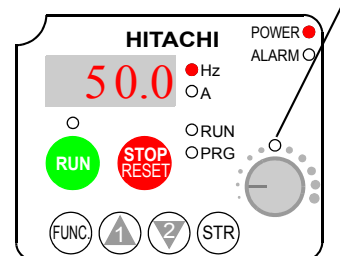
Potentiometer Aktiv LED
