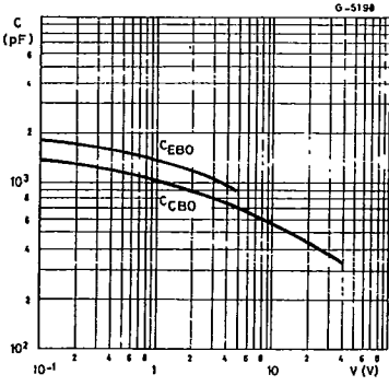
Capacitances (PNP types).
