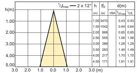
10-50W G53 AR111 WH 24D 3000K
