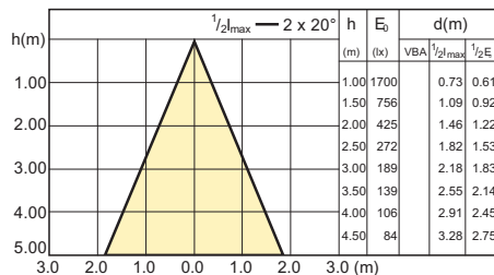
15-75W G53 AR111 WH 40D 3000K
