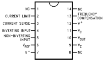
LM723CN
