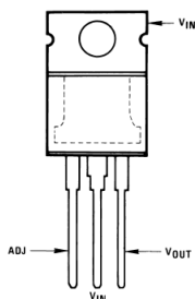
LM337T
