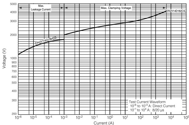
(ERZV14D182CS)
