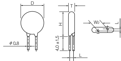
(ERZV10D182CS)
