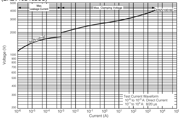
(ERZV10D182CS)
