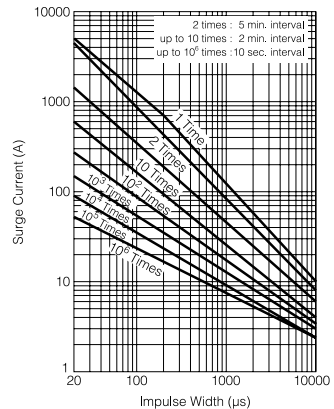
(ERZV14D182CS)
