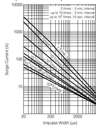
(ERZV10D182CS)
