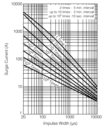
(ERZV14D182CS)
