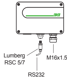
plug option C06
