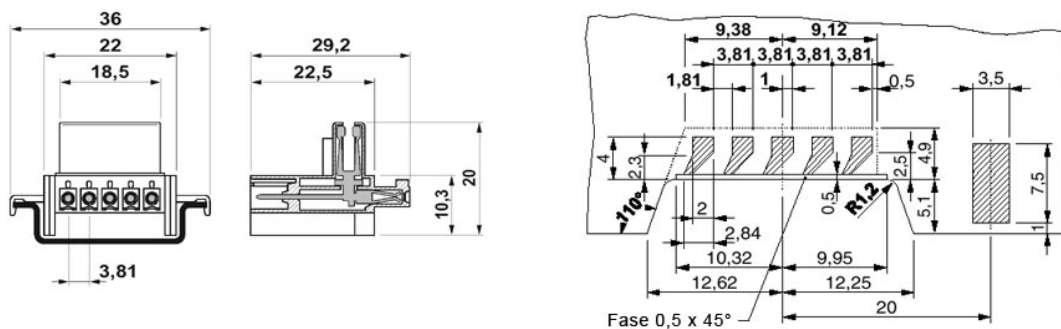
Detailmaßbild der Tragschienen-Busverbinder-Kontaktpads
