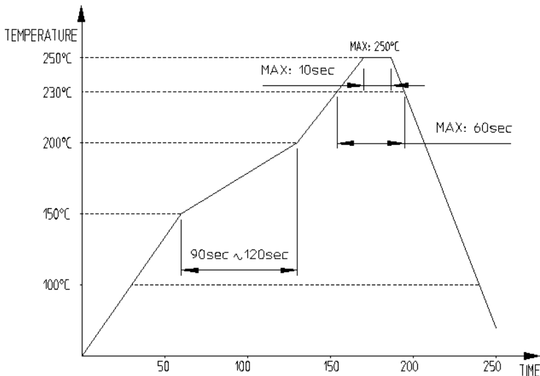
図-1 リフロープロファイル
