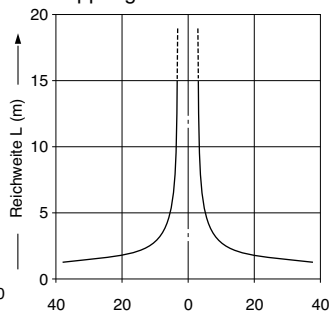
Verkippung
