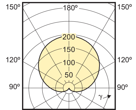
(cd/1000lm) 0°
