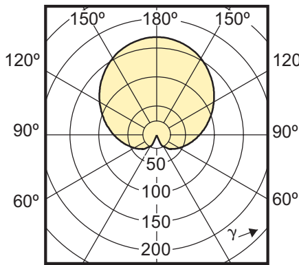
(cd/1000lm) 0°
