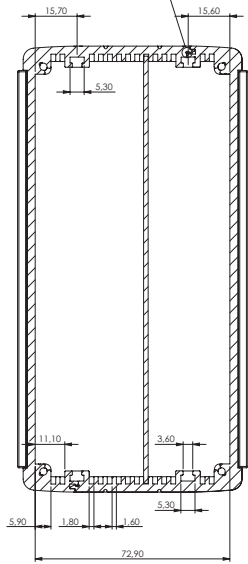
SEZIONE B-B
