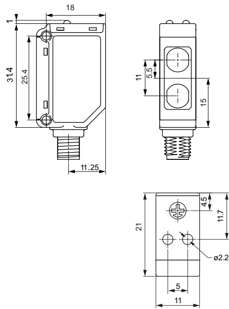
Fig. 7 Plug
