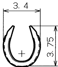
A-A sec.
