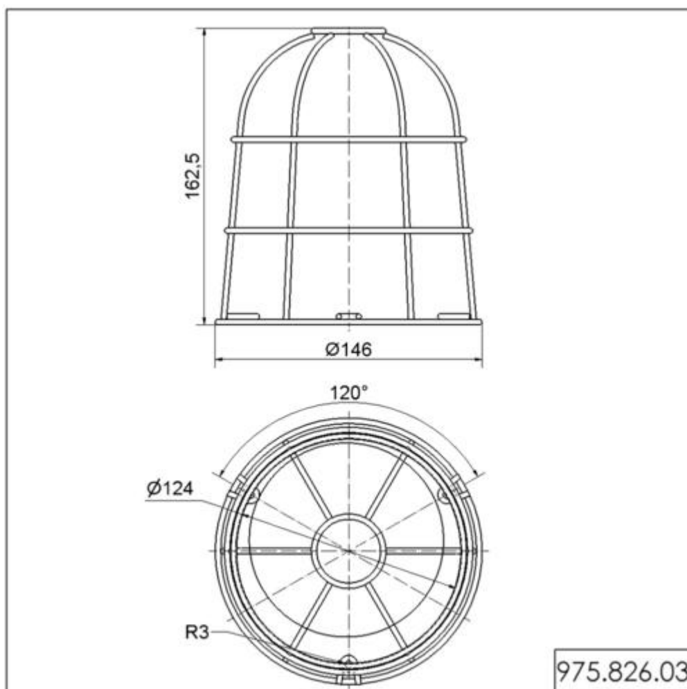
Drahtschutzkorb
