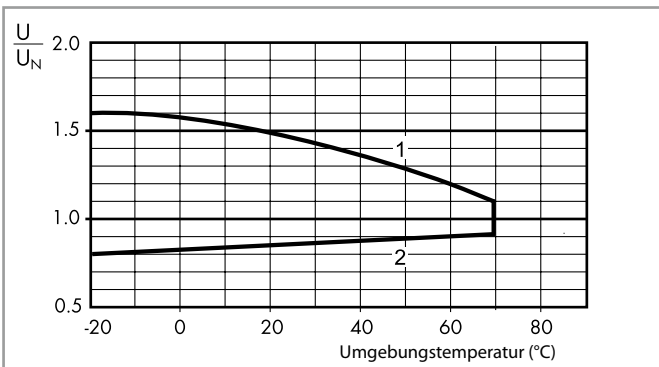
R 67 - DC Spulen-Betriebsspannungsbereich, 67.xx-4300 im Standardbetrieb (Dauerbetrieb) bei (-40...+70)°C
