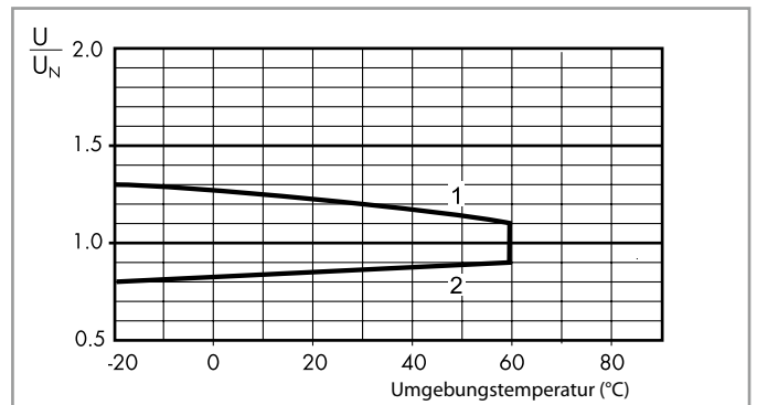
R 67 - DC Spulen-Betriebsspannungsbereich, 67.xx-4500 im Standardbetrieb (Dauerbetrieb) bei (-40...+60)°C
