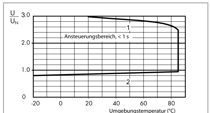
R 67 - Kurzzeitige DC Spulen-Ansteuerung, 67.xx-4300/4500 im Energiesparmodus mit Haltespannung bei (-40...+85)°C
