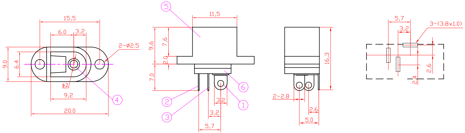
线路板安装尺寸示意图
