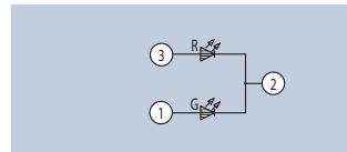
Schaltung · Circuit
