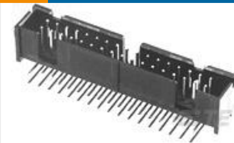
TE Part #103311-5 020 LOPRO HDR RA 30DP
