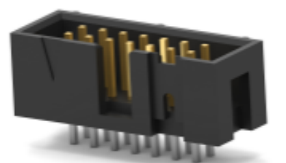
TE Part # 1761681-5 IDC LOW PRO HDR 14P VERT HT BLACK
